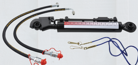
HYDRAULISK TOPPSTAG TCVHN, 620 MM KAT.2 Varenr. TCVHN356330022
