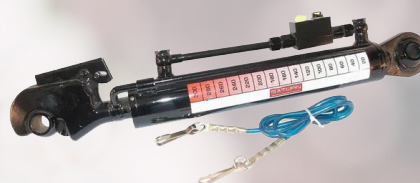
HYDRAULISK TOPPSTAG MED TILBAKESLAGSVENTIL KATEGORI 2/2 Varenr. TCVNN356330022
